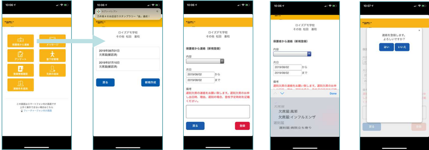
欠席・遅刻、理由、日時を選択
